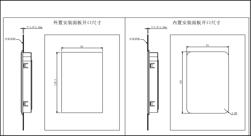
图7-12: 键盘安装开口尺寸图(尺寸单位: mm)
