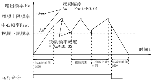
图 5-28: 摆频工作示意图
