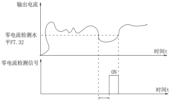
图5-21. 零电流检测示意图
