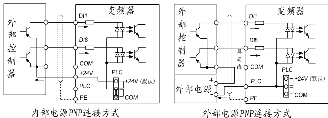
图4-15: 信号输入端子接线图--开路集电极 PNP 接线方式
