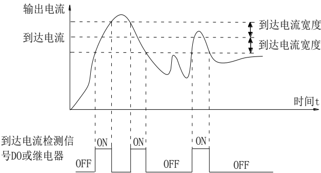
图5-23. 到达电流检测示意图
