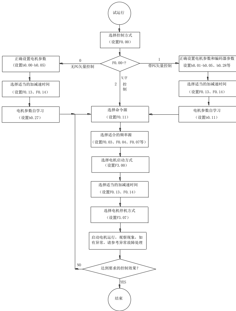
图 4-15：试运行图
