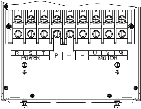
图4-6:45kW~75kW G3 主回路端子图
