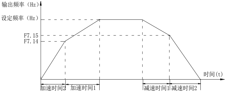
图5-16. 加减速时间切换示意图
