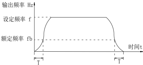
图5-9. S 曲线加减速 B 示意图
