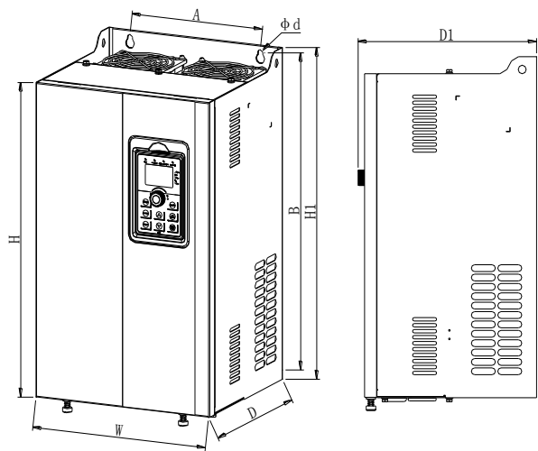
图7-4： 11kW~220kW G3 外形尺寸
