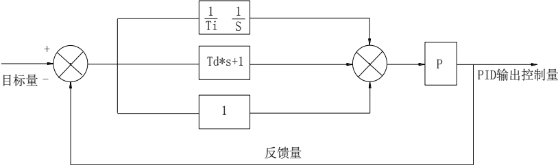
图 5-31：过程 PID 原理框图
