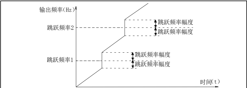
图5-15. 加减速过程中跳跃频率有效示意图
