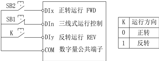
图5-6. 端子命令方式：三线制控制模式 2
