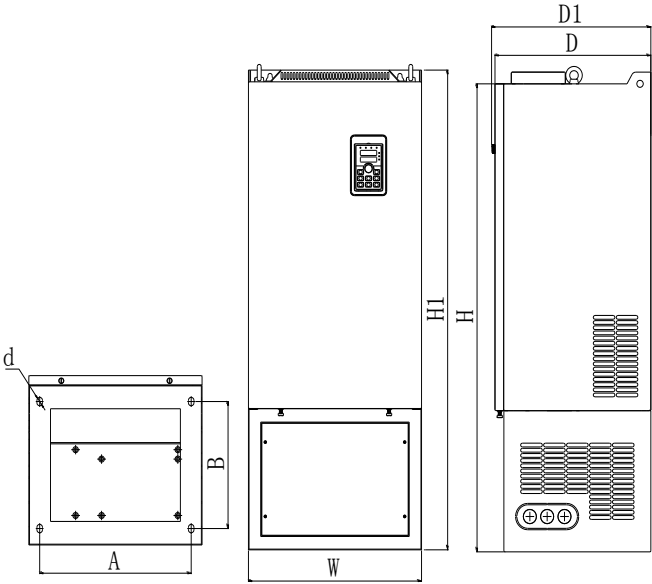
图7-7：132kW G3（带有直流电抗器底座）外形尺寸
