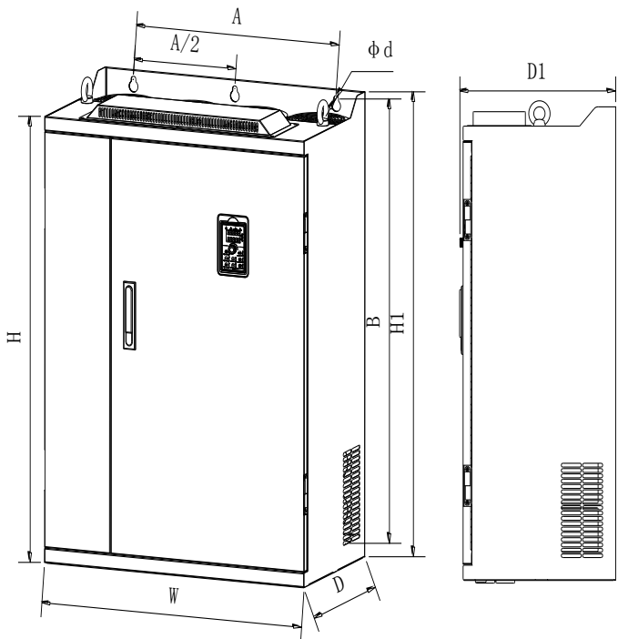
图7-5：250kW~400kW G3 外形尺寸
