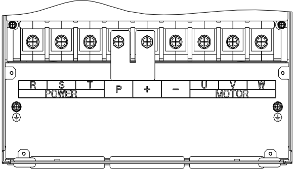
图4-7:93kW~110kW G3 主回路端子图
