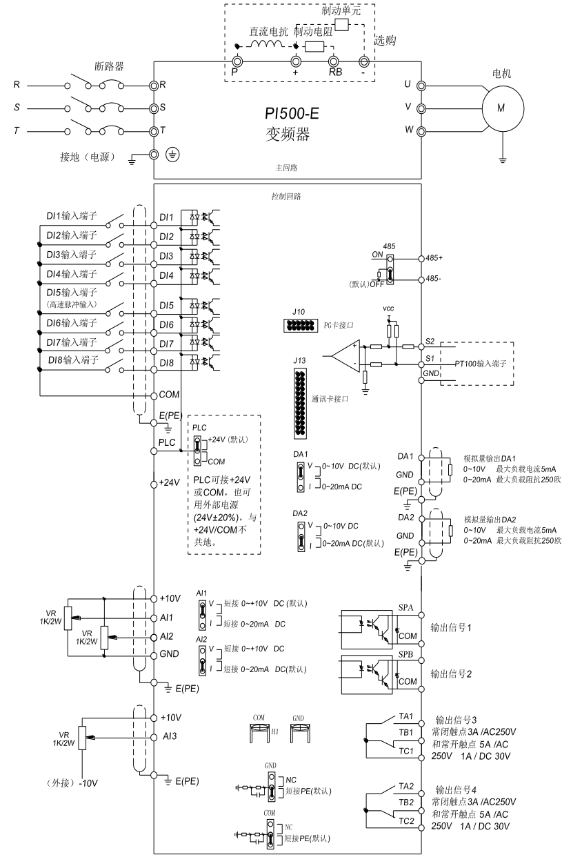
图4-3: 配线图
