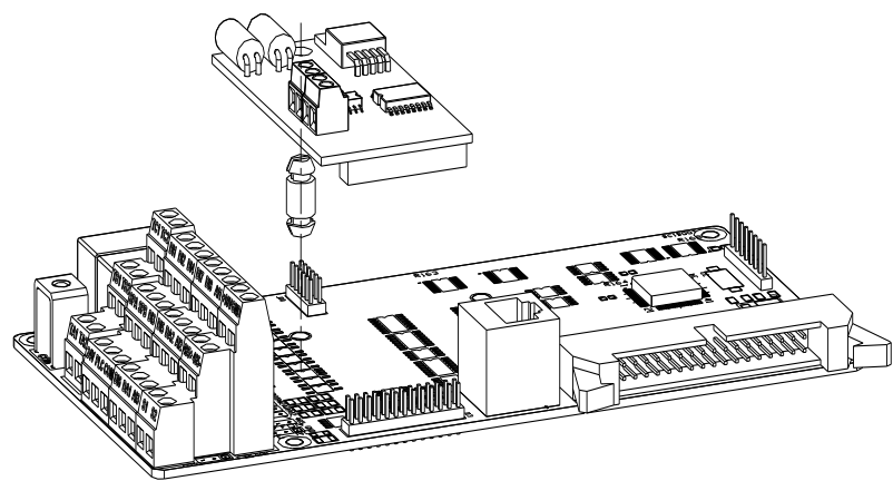
图 IV-1：CAN 总线通信卡在 PI500-E 控制板上的安装
