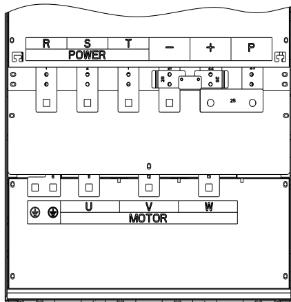
图4-9:160kW~220kW G3 主回路端子
