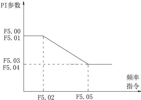
图5-10. PI 参数示意图
