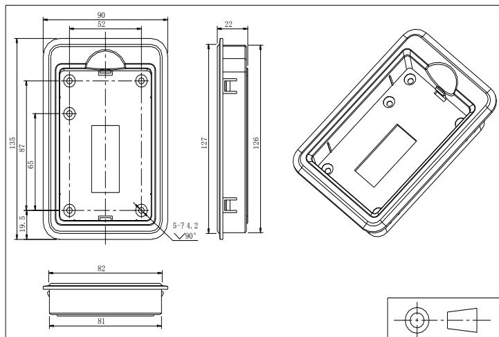
图7-11: 键盘仓尺寸图(尺寸单位: mm)
