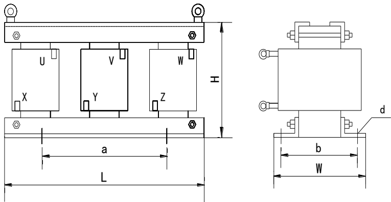
图 9-2: 交流输入电抗器外形尺寸图
