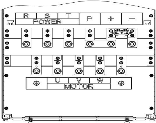
图4-8:132kW G3 主回路端子
