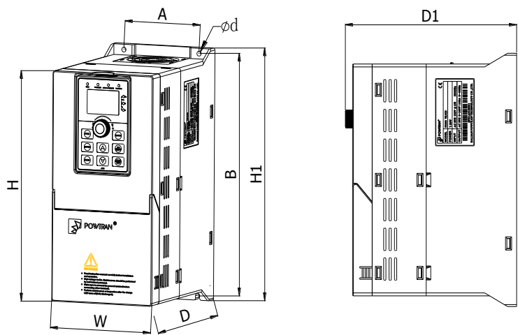
图7-3： 5.5kW~7.5kW G3 外形尺寸
