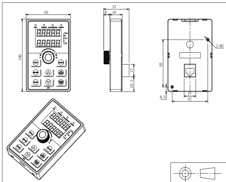
图7-10: PI500-E 键盘尺寸图(尺寸单位: mm)
