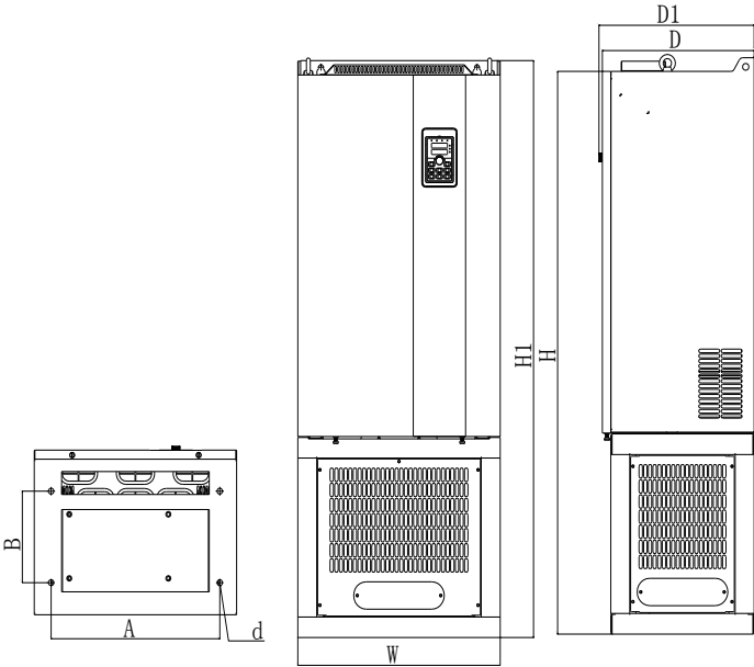
图7-8：160kW~220kW G3（带有直流电抗器底座）外形尺寸
