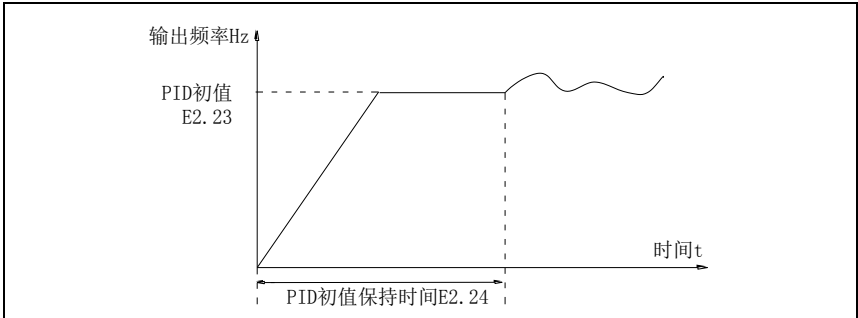
图 5-33: PID 初值功能示意图
