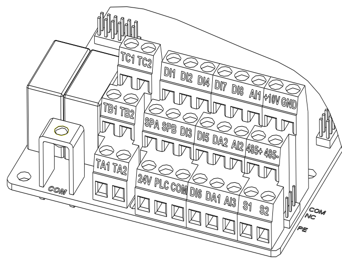
图4-12:控制板控制回路端子
