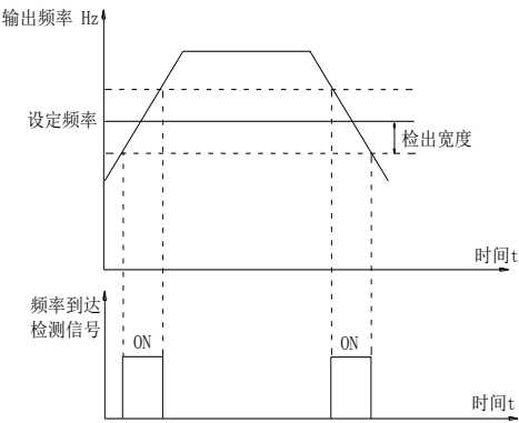
图5-19. 频率到达 频率到达检出幅值示意图 检出幅值示意图
