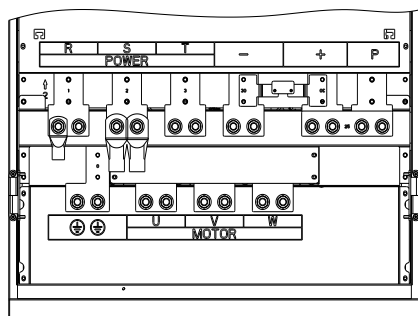
图4-10:250kW~400kW G3 主回路端子
