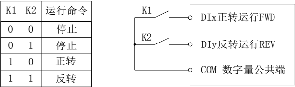
图5-4. 端子命令方式：两线制模式 2
