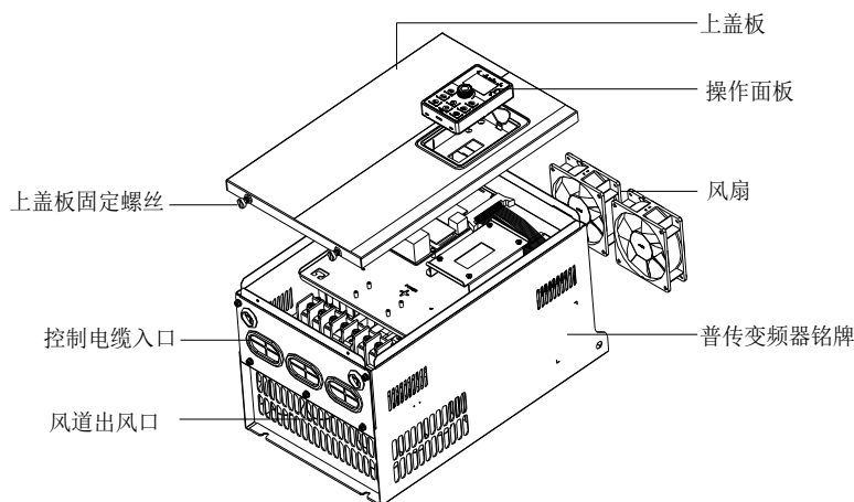
图7-1: 11kW G3 以上产品外型图、安装孔位尺寸
