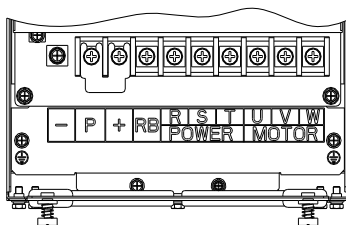
图4-4:18.5kW~22kW G3 主回路端子图
