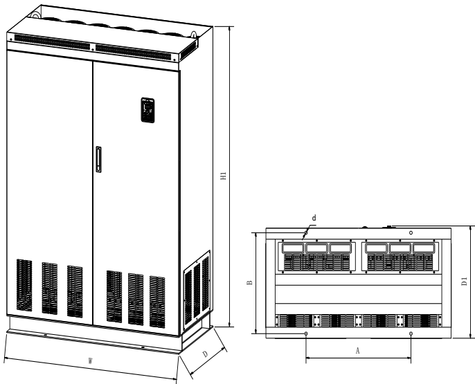
图7-6：450kW G3 外形尺寸
