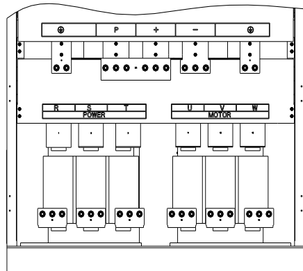
图4-11:450kW G3 主回路端子
