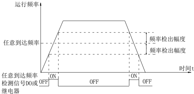
图5-20. 任意到达频率检测示意图
