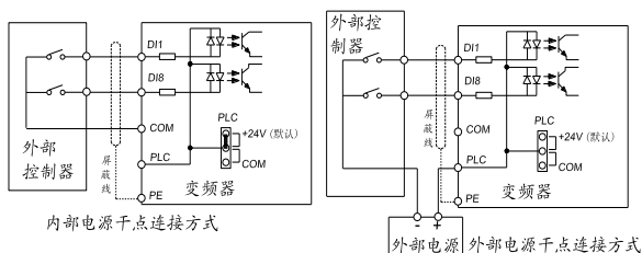
图4-13: 信号输入端子接线图--干接点方式
