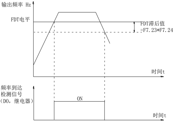
图5-18. FDT 电平示意图
