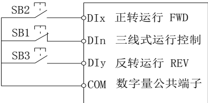
图5-5. 端子命令方式：三线制控制模式 1
