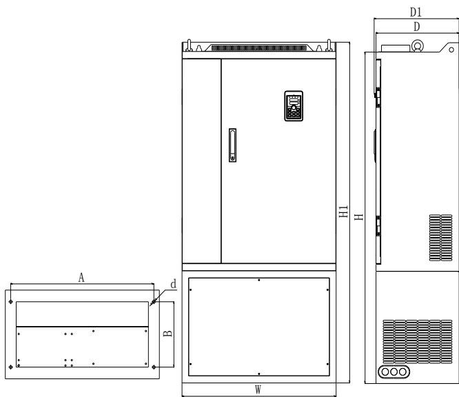
图7-9：250kW～400kW G3（带有直流电抗器底座）外形尺寸
