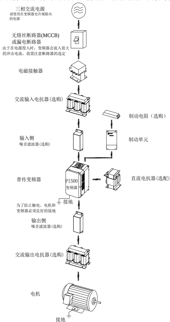
图 9-1：选件接线图
