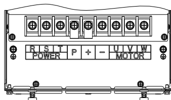
图4-5:30kW~37kW G3 主回路端子图
