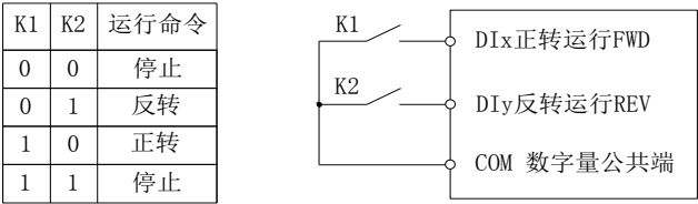
图5-3. 端子命令方式：两线制模式 1
