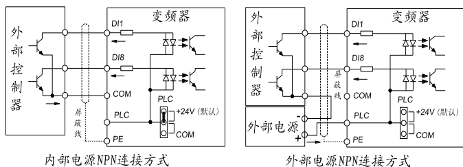
图4-14: 信号输入端子接线图--开路集电极 NPN 接线方式
