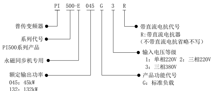
图 1-2：型号说明
