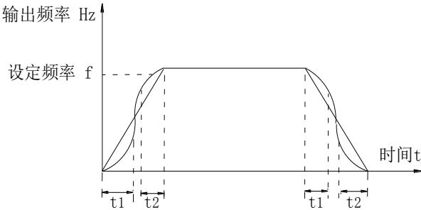
图5-8.：S 曲线加减速 A 示意图
