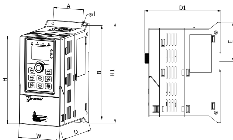
图7-2: 0.75~4kW G3 外形尺寸
