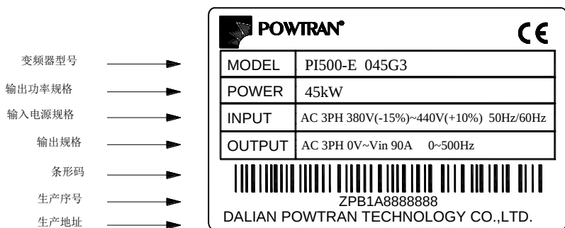
图 1-1：铭牌说明
