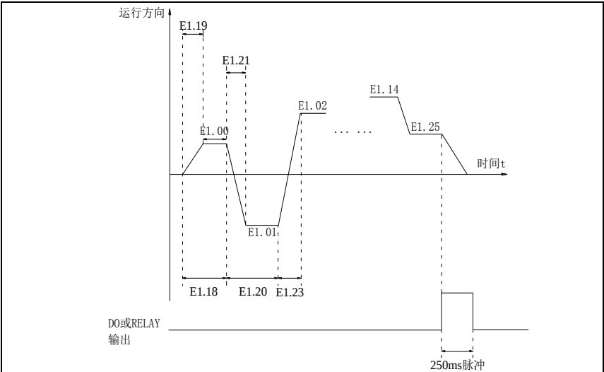
图 5-30：简易 PLC 示意图 变频器完成一个循环后，自动开始进行下一个循环，直到有停机命令时停止。
