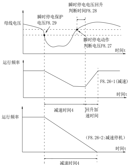
图5-24. 瞬时停电动作示意图
