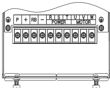
图4-3:11kW~15kW G3 主回路端子图
