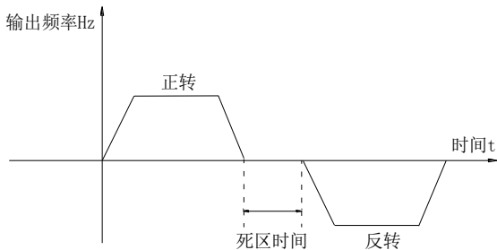
图5-17. 正反转死区时间示意图
