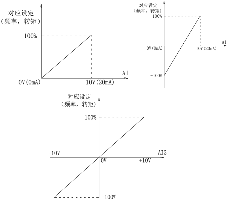
图5-7. 模拟给定与设定量的对应关系
